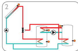
2-Speicher-Solarsystem mit Ventillogik und Wärmeaustauschregelung (Seite 11)
