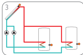
2-Speicher-Solarsystem mit Pumpenlogik (Seite 14)
