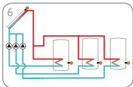
3-Speicher-Solarsystem mit Pumpenlogik und Vorranglogik (Seite 23)
