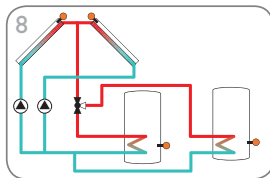
Solarsystem mit Ost-/Westdach und 2 Speichern (Seite 29)
