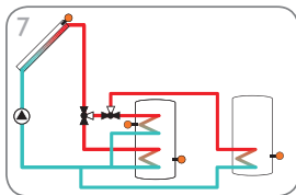
Solarsystem mit Schichtspeicher und 2. Speicher (Seite 26)
