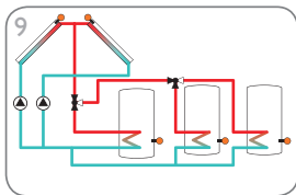
3-Speicher-Solarsystem mit Ost-/Westdach (Seite 32)
