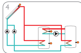
2-Speicher-Solarsystem mit Pumpenlogik und Wärmeaustauschregelung (Seite 17)
