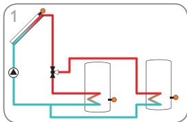
2-Speicher-Solarsystem mit Ventillogik, 1 Pumpe, 3 Sensoren und 3-Wege-Ventil (Seite 8)
