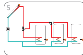
3-Speicher-Solarsystem mit Ventillogik und Vorranglogik (Seite 20)
